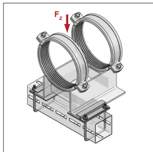
Set Piastra a Z CENTUM® per supporti scorrevoli e slitte di scorrimento con larghezza da 140 mm
