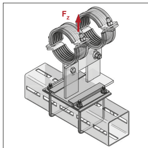
Set Piastra a Z CENTUM® per supporti scorrevoli e slitte di scorrimento con larghezza di 100 mm
