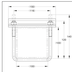
U-bolt 120 / 140 M10
