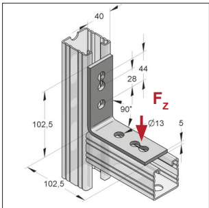
Angolare per binari 40/5 4-fori 90°
