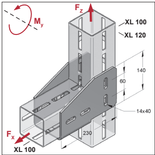
Squadretta XL 100
