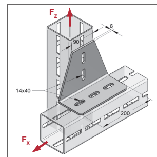
Piastra a T ad angolo CENTUM®
