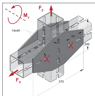
Piastra a croce da XL 100 CENTUM
