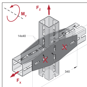
Piastra a croce XL 80 CENTUM
