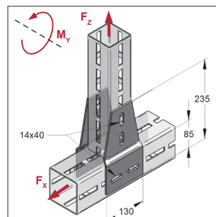
Piastra a T con lembo piegato CENTUM®
