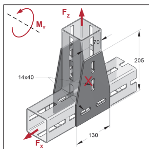
Piastra a T XL 80 CENTUM®
