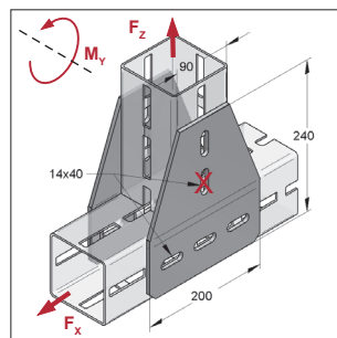
Piastra a T da XL 100 CENTUM®
